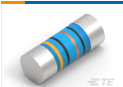
TE 产品编号2-2176316-4 MELF SMA_A 8K2 0.1% 15PPM 0207 1W
