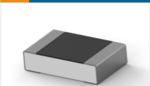
TE 产品编号1-2176374-0 RQ 0805 133R 0.1% 10PPM 1K RL
