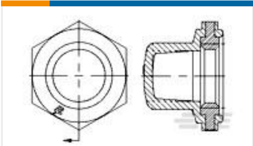
TE 产品编号1274595-1 JACK, VERTICAL, PCB, HIGH TORQUE, MINI B
