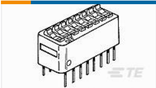
TE 产品编号 3-435640-8 DIP SW 7 POSN SEALED
