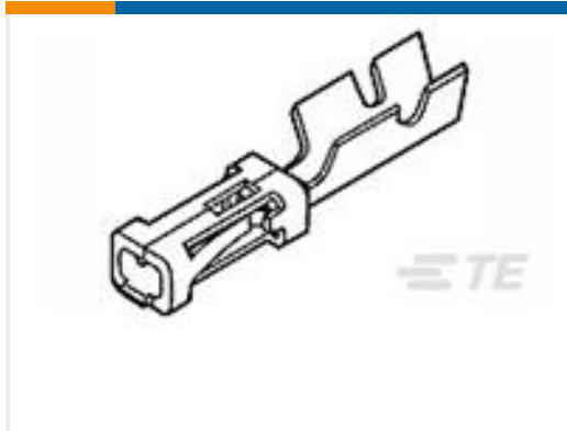
TE 产品编号167301-4 MOD-4 REC.CONT.SCP
