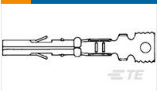
TE 产品编号794001-2 MR RECPT AU PHBZ LP 26-24
