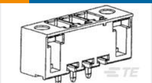
TE 产品编号796867-3 3 POS TERMI-BLOK HDR VERTICAL
