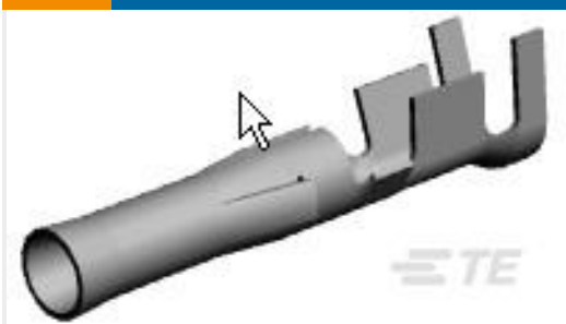
TE 产品编号350415-1 .093 COMM P&S SOK 14-20 PTPBR
