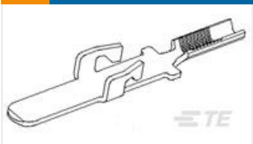
TE 产品编号1217072-1 CONT AMVAR 125 BLADE 020 TPBR
