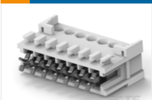
TE 产品编号1-2232892-7 7P MONOPLUG 2.5
