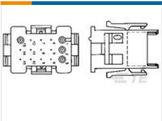
TE 产品编号1-640513-0 15P MR II CAP HSG V0 RED
