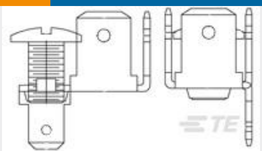
TE 产品编号157431-1 250 FASTON, TAB ASSY, BR
