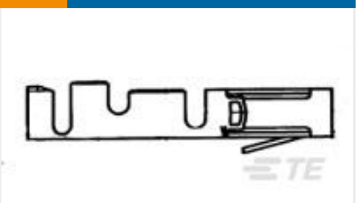
TE 产品编号141098-6 MOD-4 REC.CONTACT
