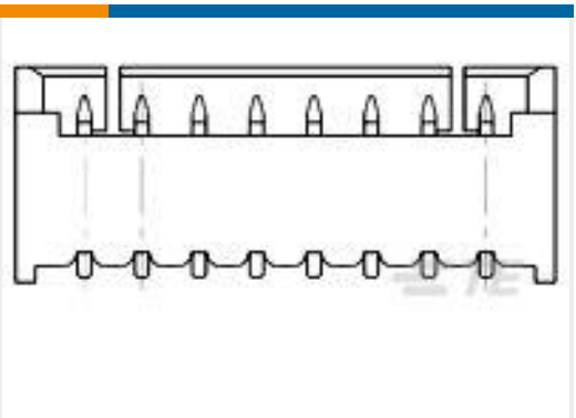
TE 产品编号1734829-4 1.25 WTB HDR DIP, 4 POS
