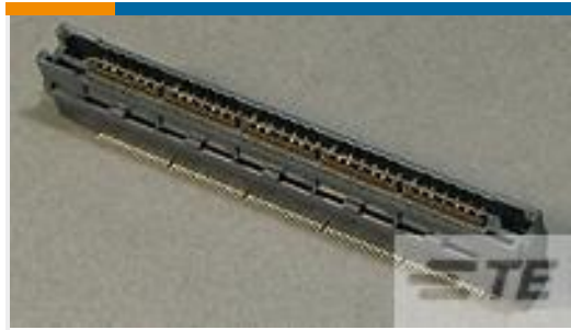
TE 产品编号 767178-5 MICTOR RAISED VERT RECPT ASSY,
