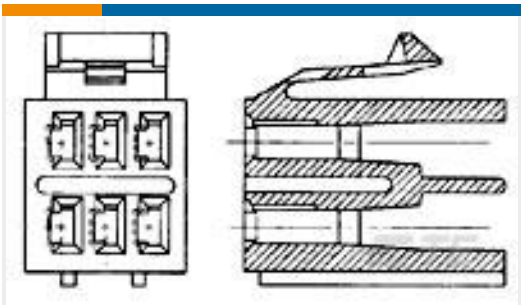
TE 产品编号1-962349-1 6P STIFT-GEH 3MM
