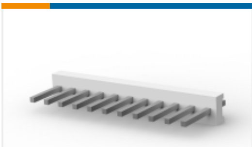
TE 产品编号 1-640383-1 11P MTA156 HDR ASSY STR SQ SN
