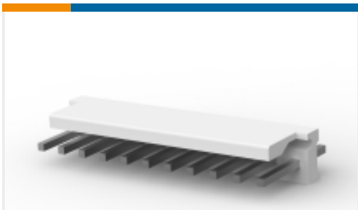
TE 产品编号 1-644752-1 11P MTA156 HDR ASSY SQ STR F/L
