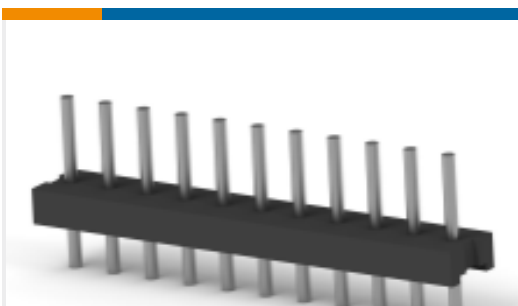
TE 产品编号 1-644750-1 11P MTA156 HDR ASSY STR RND SN
