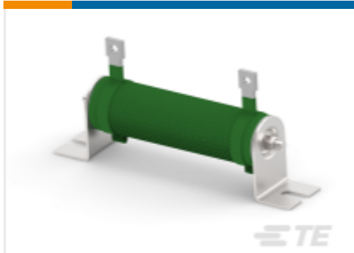
TE 产品编号2-1879451-5 线绕电阻器：矿物，2.5 Kw
