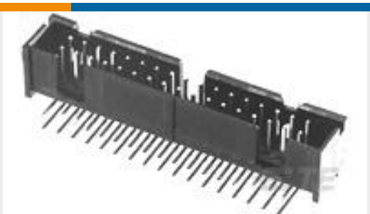
TE 产品编号 1-103311-0 050 LOPRO HDR RA 30DP
