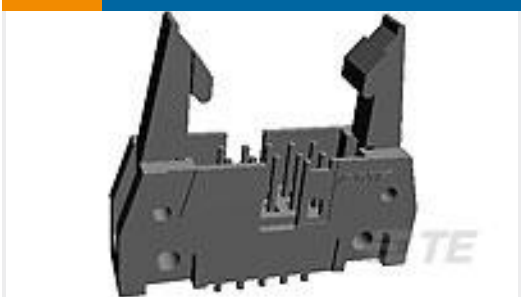
TE 产品编号5111824-9 A/L UNIV HDR 39/40P VERT LG LAT
