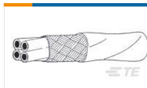
TE 产品编号3825243001 44A1141-20-0/2/6/9-9
