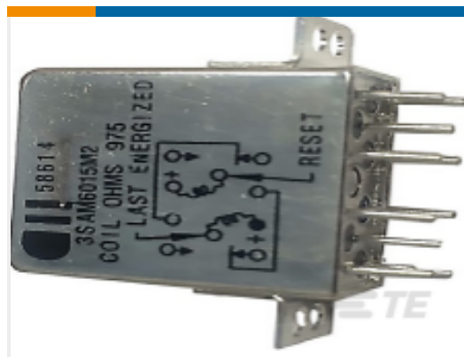
TE 产品编号 1-1617522-6 3SAM1819A2=M39016/32-001
