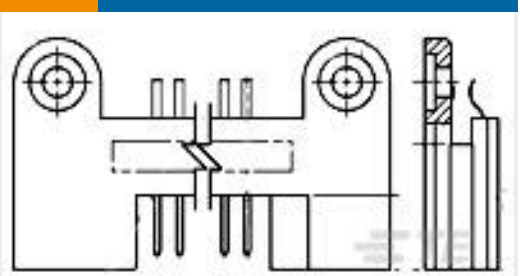
TE 产品编号530785-2 BOX PIN 150 POS 075 C/L
