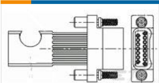
TE 产品编号260297-000 D-181-1224-90/9CS554
