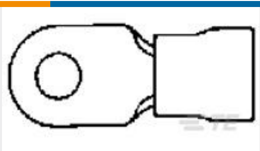
TE 产品编号53944-1 TERMINAL,R PVF2 PG 8 3/8
