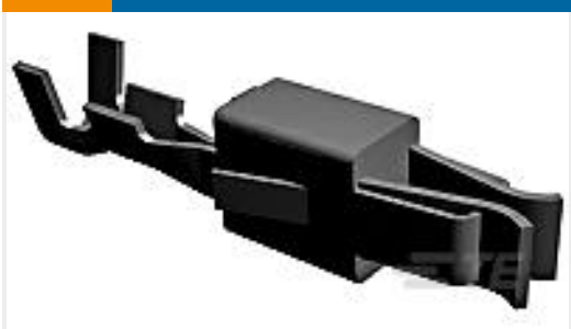
TE 产品编号2-927774-1 JPT REC 2.8 Contact SRC Au
