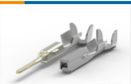
TE 产品编号2109005-1 MULTILOCK，母端和公端
