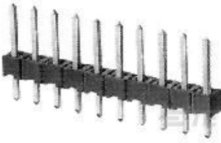
TE 产品编号1-826646-3 13P AMPMODU II STIFT LEI
