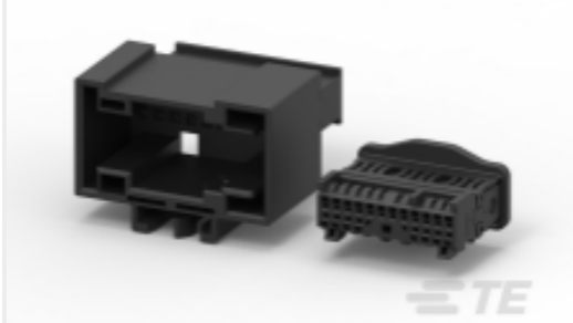
TE 产品编号1473244-1 MQS , 连接器壳体
