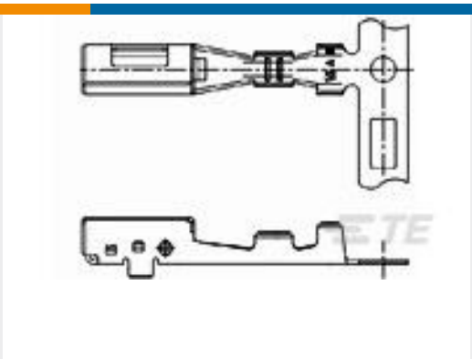
TE 产品编号1743656-1 090III MLC REC(L) CONT
