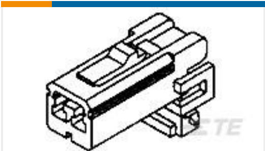
TE 产品编号776128-6 2POS .070 MULTILOCK PLUG LEFT
