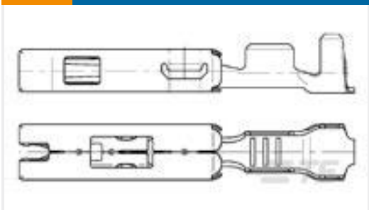
TE 产品编号929025-1 1.5MM SFC
