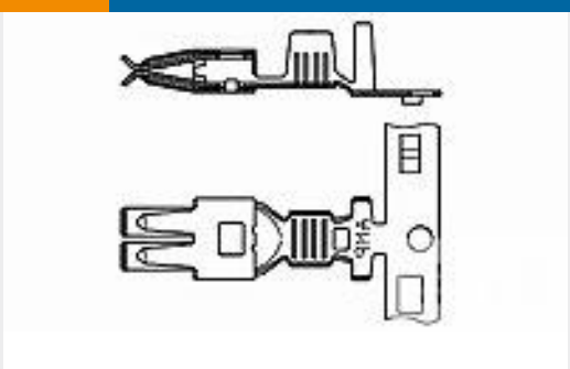
TE 产品编号963894-1 STECKHUELSE 6,3
