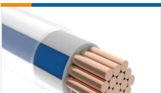
TE 产品编号9968783001 ACW0219-0.50-79(NS)
