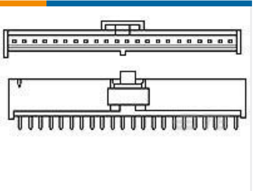
TE 产品编号1888291-1 FPH-0421G=FLXPAC HDR P 04 ST LF
