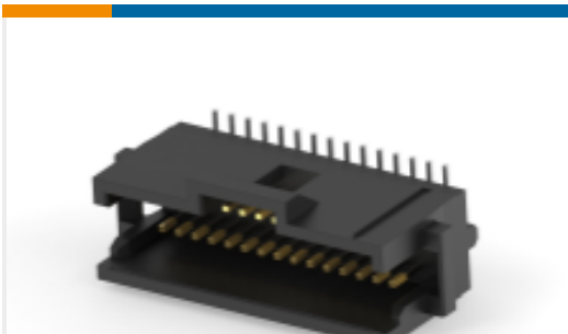
TE 产品编号3-1825601-0 30 SYS50 SMT HDR DR SHD W/O CAP
