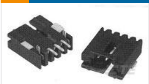
TE 产品编号 58336-1 HEAD (IDC) MODU MTE W/O TL
