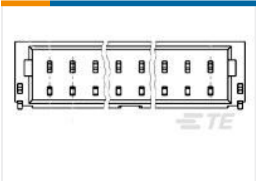
TE 产品编号1734709-2 1.0 WTB HDR SR RA 2 POS
