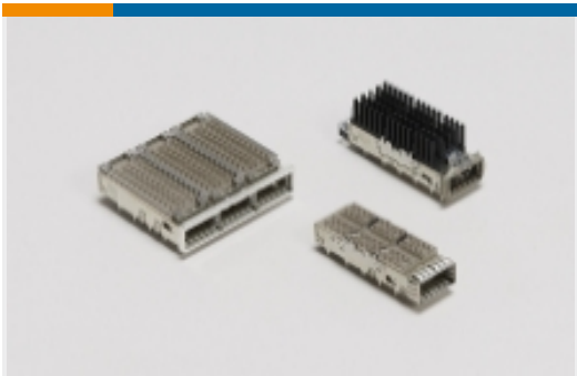
QSFP/QSFP+/zQSFP+(168)
