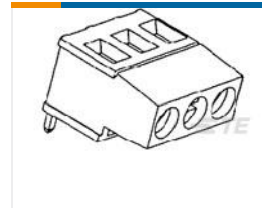
TE 产品编号1546073-3 3 POS 5.08MM TERMI-BLOK
