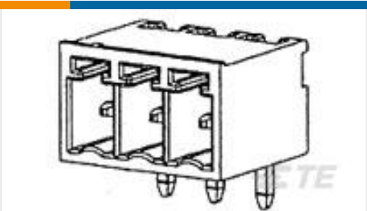
TE 产品编号1-284512-2 12 POS TERMI-BLOK HDR 900 POLA
