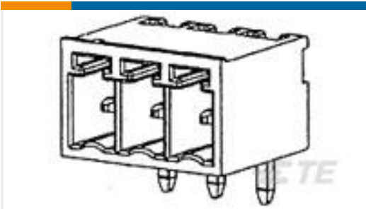
TE 产品编号1-284512-0 10 POS TERMI-BLOK HDR 900 POLA
