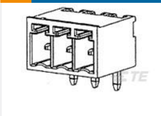
TE 产品编号1-284512-2 12 POS TERMI-BLOK HDR 900 POLA
