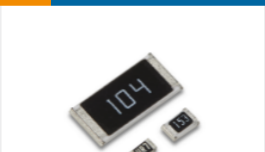
TE 产品编号2-2176345-1 CRGCO 1210 470R 1%
