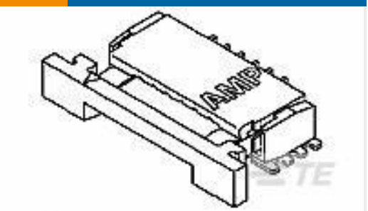
TE 产品编号1-84952-2 1MM FPC HORZ.BTTM CONT.ASS.12P
