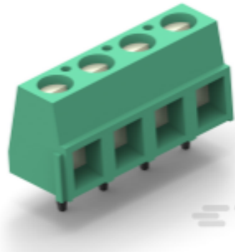
TE 产品编号 282837-4 TERMI-BLOK PCB MOUNT 4P
