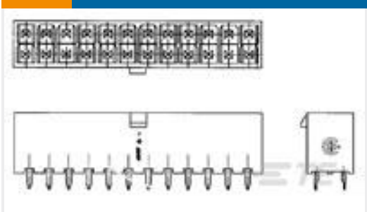
TE 产品编号1586037-8 8P VERT HDR VAL-U-LOK V2
