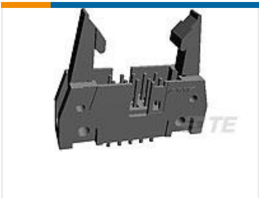
TE 产品编号102321-6 026 UNIV HDR SP 4S 30DP STD L1
