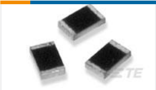
TE 产品编号1-1625867-4 RP 1J 0.166W 1K65 0.1% 25PPM 1K RL
