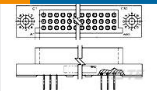
TE 产品编号532786-5 3 ROW BOX RECP 165 POS 100 C/L
