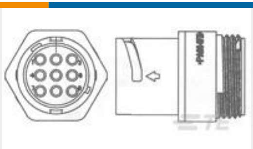
TE 产品编号1445826-3 REC,11-8,FRE HNG,LG INS,STD KE
