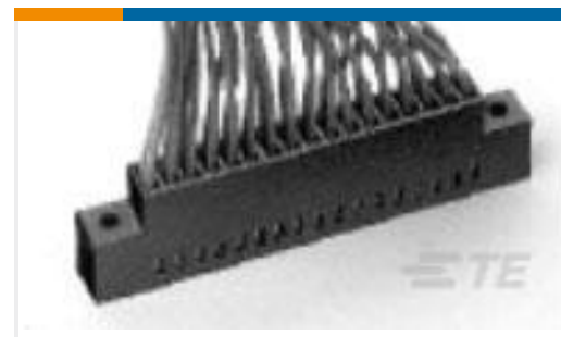
TE 产品编号1-86264-7 26 MODIV HSG COMP DR .100 EARS
